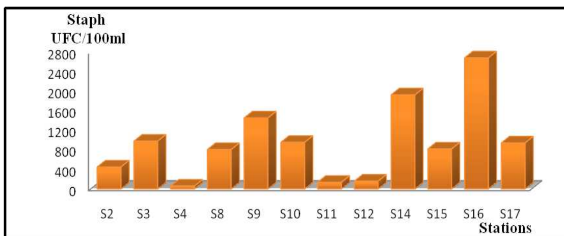
Figure III.25. Variations des concentrations moyennes des Staphylocoques (Staph) en fonction des stations.
