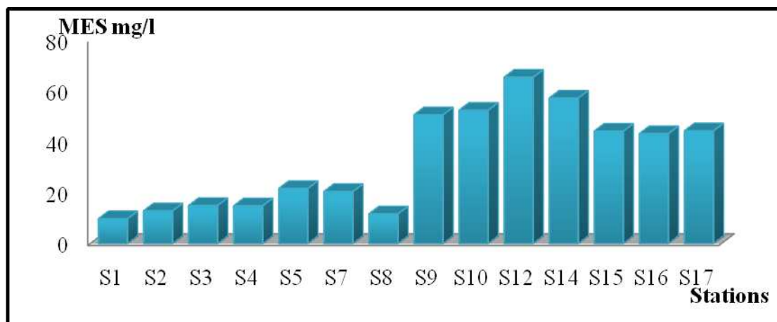
Figure III.10. Variation des moyennes de MES en fonction des stations.
