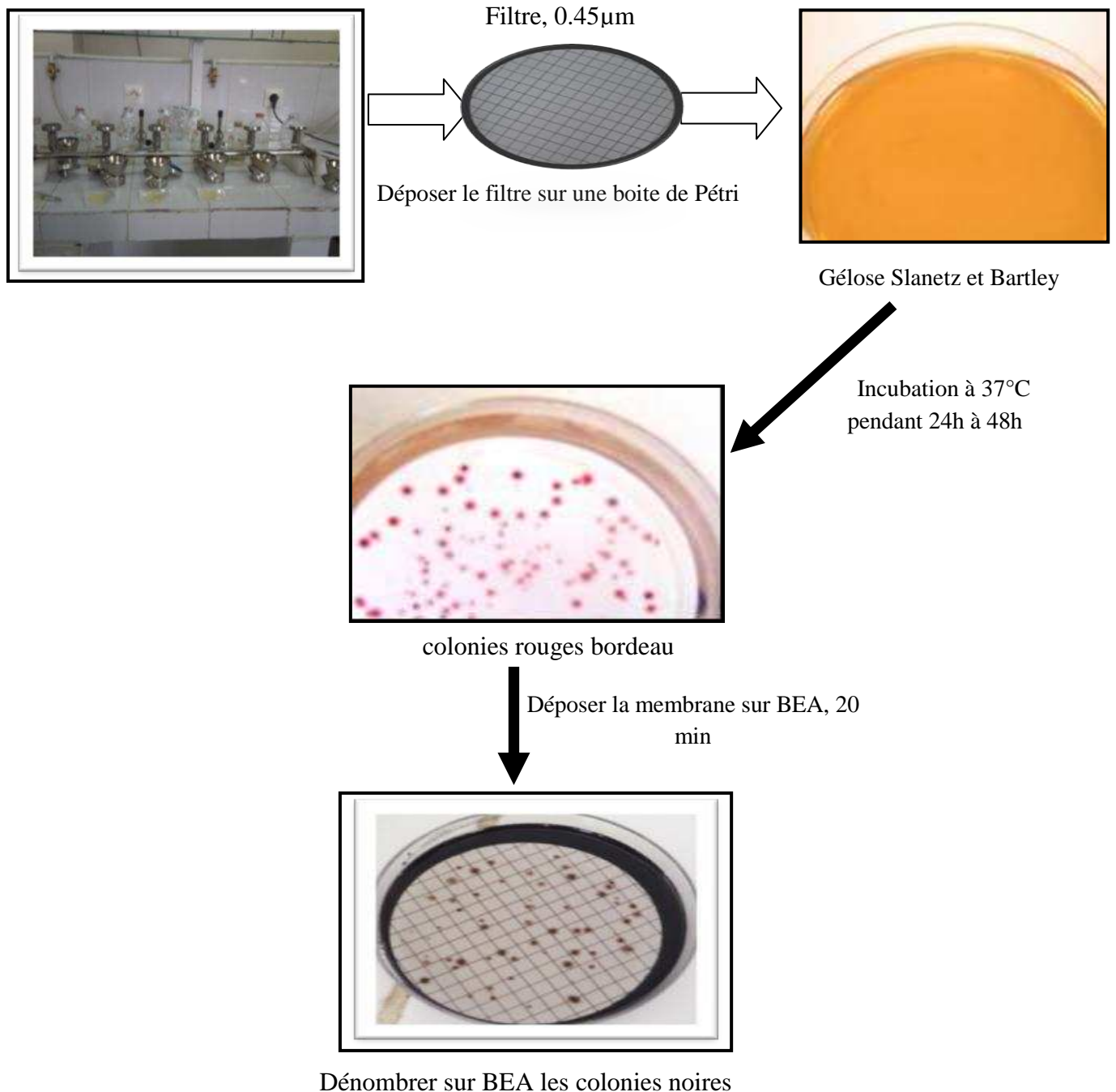
Figure II.14: Technique de dénombrement des streptocoques fécaux.
