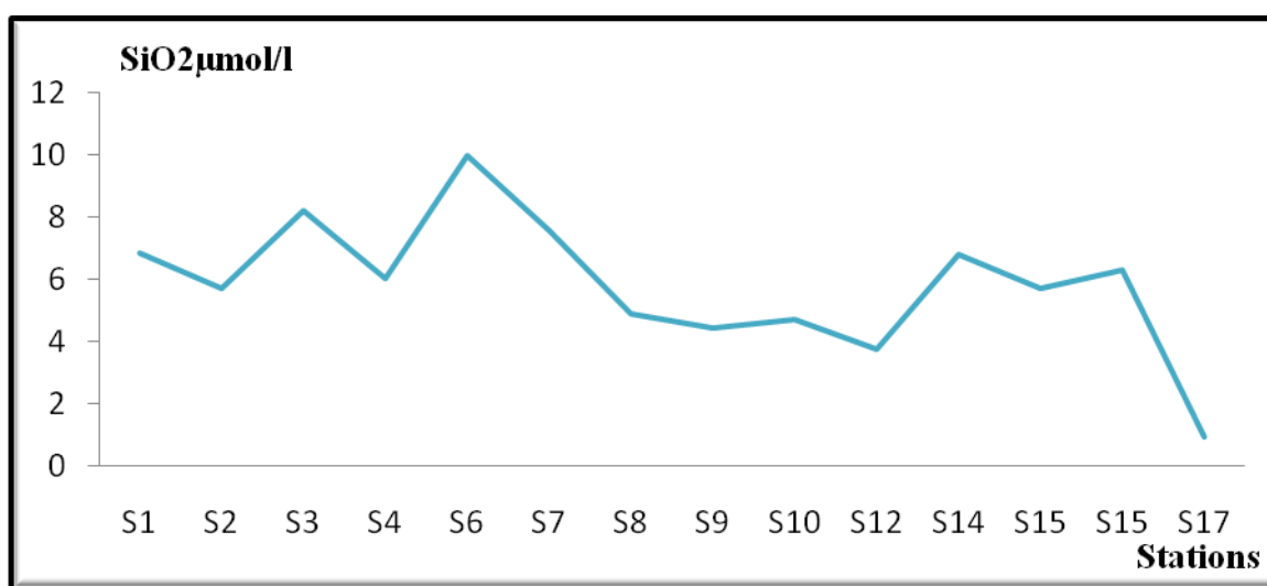
Figure III.19. Variations des concentrations moyennes des silicates en fonction des stations
