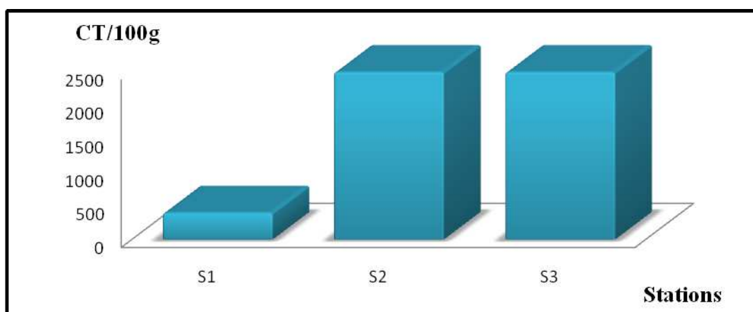
Figure III.28. Variations des concentrations des coliformes totaux (CT) dans les sédiments en fonction des stations.
